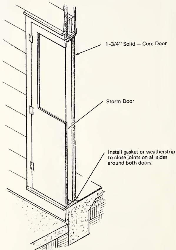
Fig. 5-4. DOOR MODIFICATIONS
