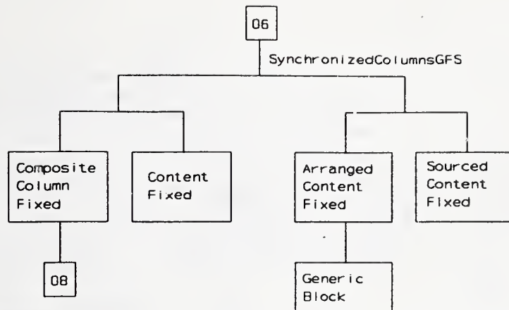
Figure 40 — SynchronizedColumns
