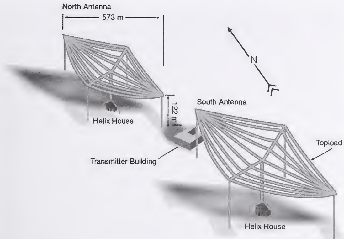
Figure 1.19. WWVB antennas.
