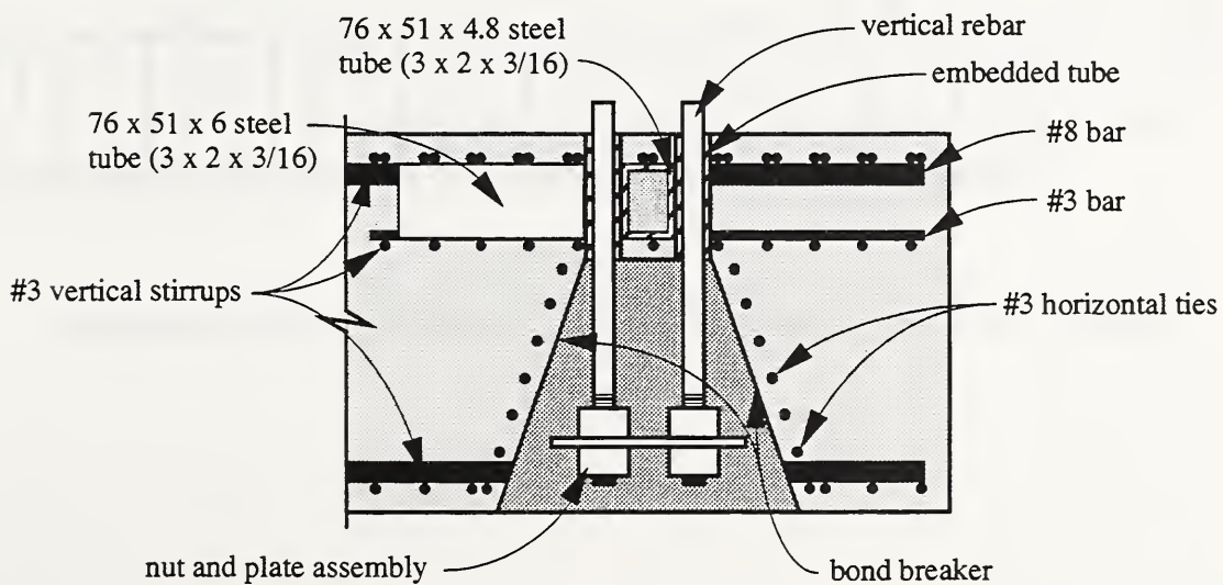
c) Section D-D
