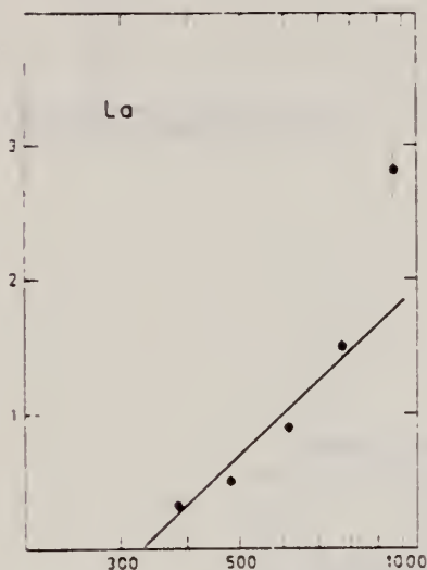
Fig. 1b. Bremsstrahlung energy (MeV)
