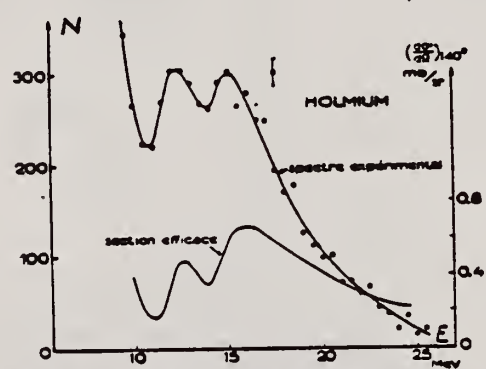
Fig. 1. Résultats expérimentaux et sections efficaces de diffusion déduites pour l'holmium. E_n = 27 \text{ MeV} .
