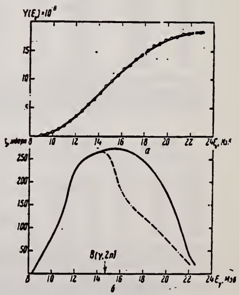
Рис. 12. а - Выход фотонейтронов для Tb; б - \sigma_n(E_{\gamma}) для Tb
