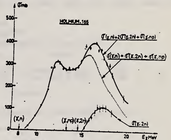
Fig. 2. — Sections efficaces de photoproduction de neutrons de 165 Ho mesurées dans ce travail.
