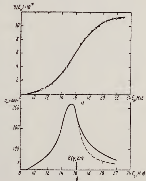
Рис. 10. а — Выход фотонейтронов для La; б — \sigma_n(E_{\gamma}) и B(\gamma, 2n) для La
