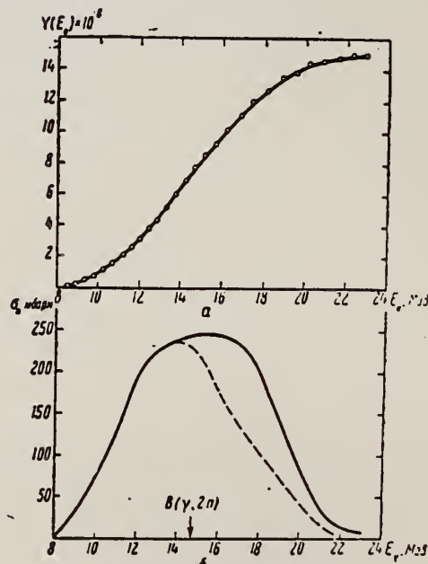
Рис. 14. а — Выход фотонейтронов для Tm; б — \sigma_n(E_\gamma) в \sigma_c(\gamma) для Tm
