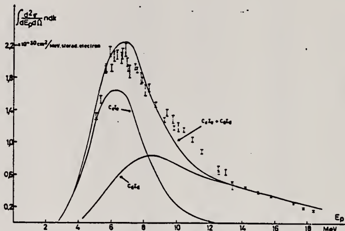
FIG. 2. — Distribution d'énergie. E_0 = 40 MeV, \theta = 75^\circ . C_e I_e = distribution des protons évaporés. C_e I_e = distribution des protons directs.
