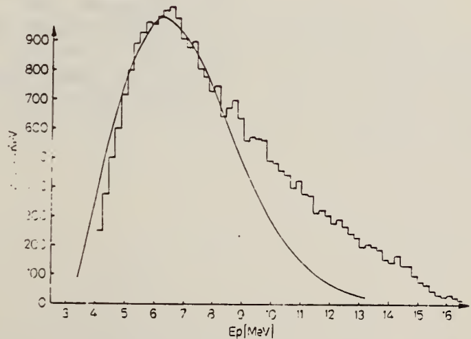
Fig. 11. Energieverteilung der Photoprotonen aus 84 Kr für E 0 = 32,5 MeV. Kurve: Berechnetes Verdampfungsspektrum
