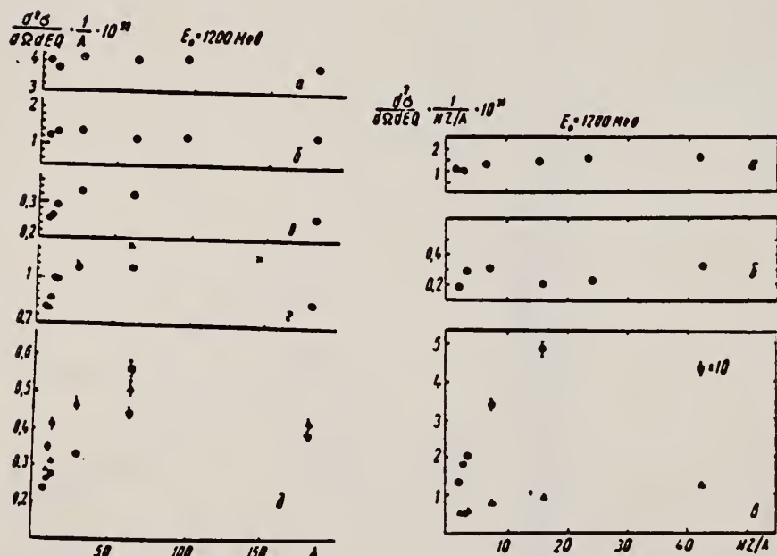
Рис. 1. Залежність перерізу (\gamma, p) -реакції від A : a - \phi = 30^\circ , E_p = 97 Mev; b - E_p = 205 Mev; c - \phi = 60^\circ , E_p = 230 Mev; z - E_p = 157 Mev ( \times - дані [3]); d - \phi = 120^\circ , \circ - E_p = 120 Mev, \Delta - E_p = 157 Mev, \square - E_p = 230 Mev. Абсолютне значення перерізу наведено при енергії протонів E_p = 120 Mev. Інші дані нормовані до перерізу для \text{Li}^7 при E_p = 120 Mev.
