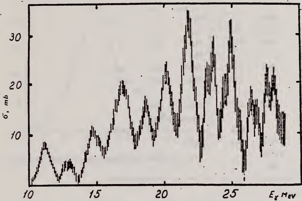
Фиг. 8. Сечение реакции \gamma^{89} (v.n).
