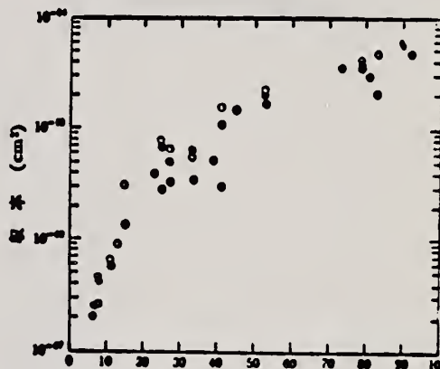
原子番号 ●: 実験値, ⊕: Johns ら, ⊙: Nathans ら, ○: Montalbetti ら 図4 ( \gamma, n )反応の収率の比較
