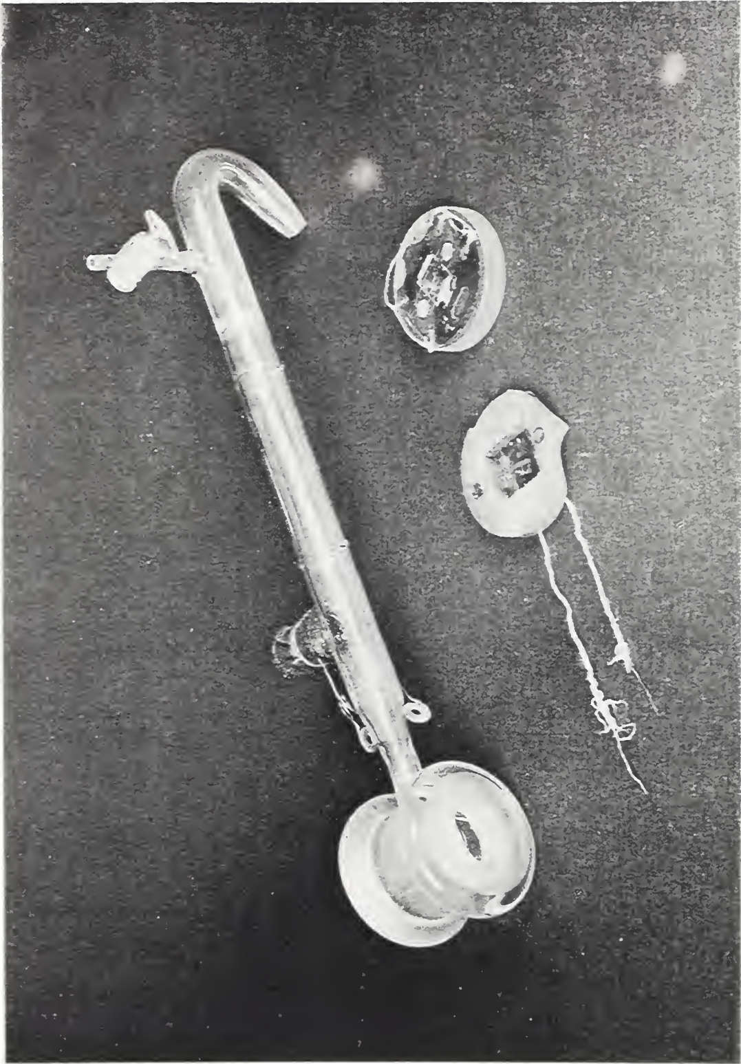
Thermopiles (1923) M202
