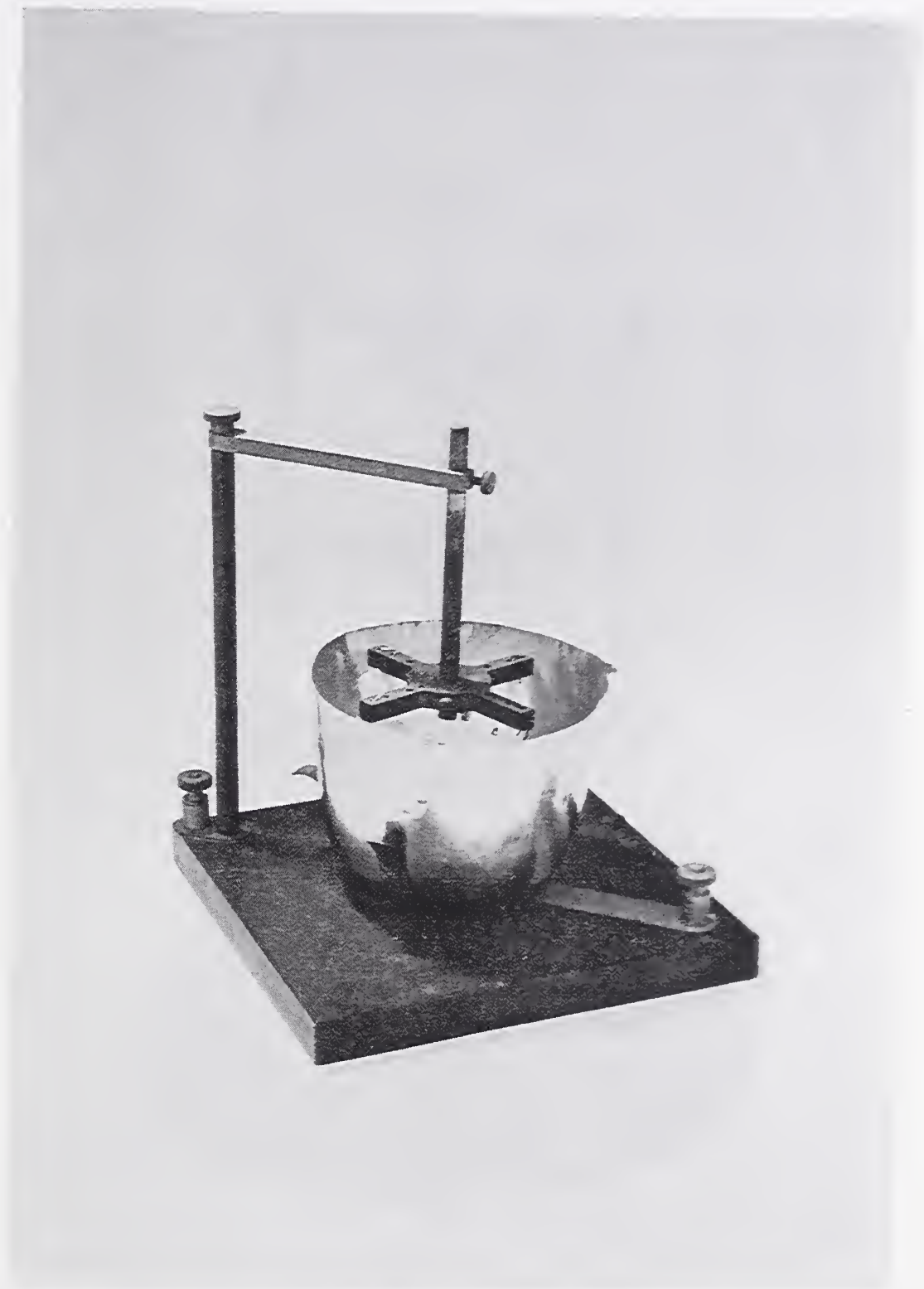
Coulometer, Rayleigh (England) (1884) M172
