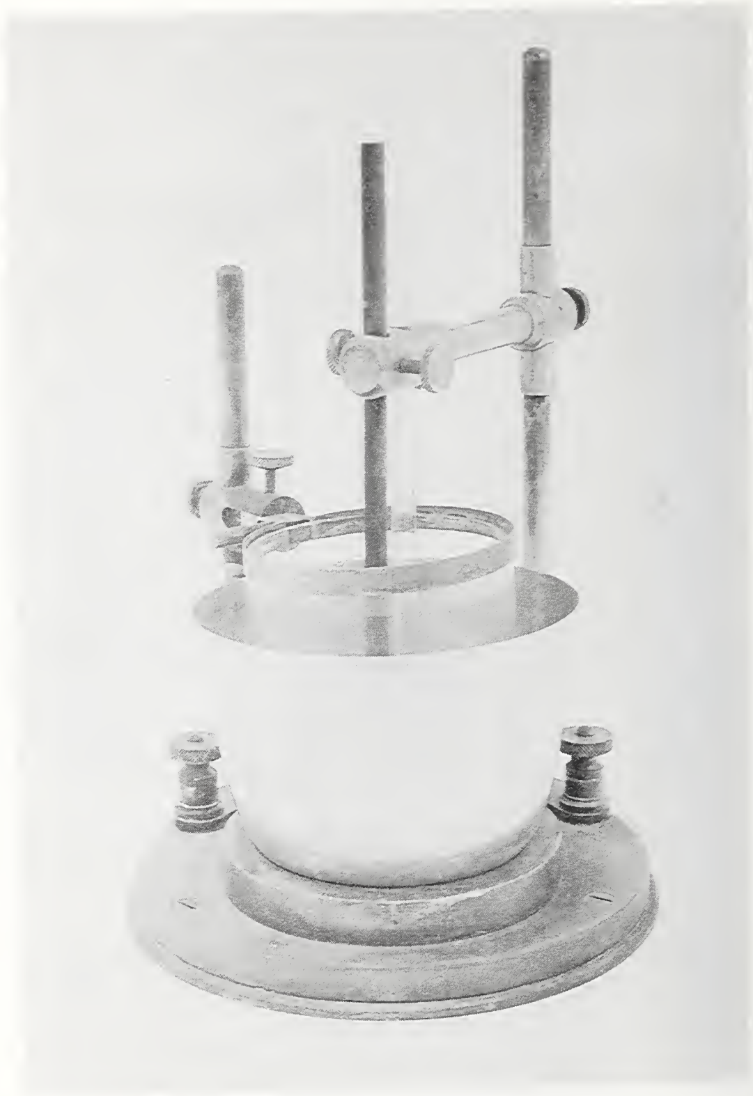
Coulometer, Smith (England) (1910) M171
